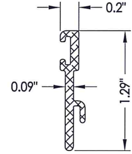
15 SILL RISER
