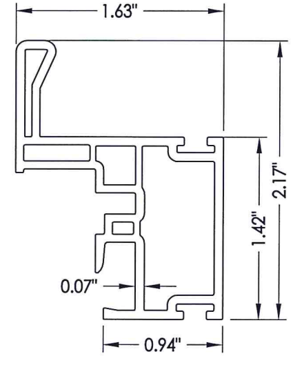
8 HANDLE STILE
