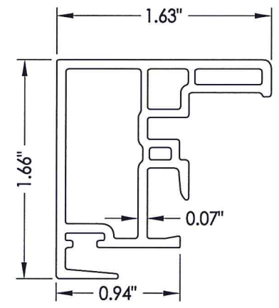
7 LOCK STILE
